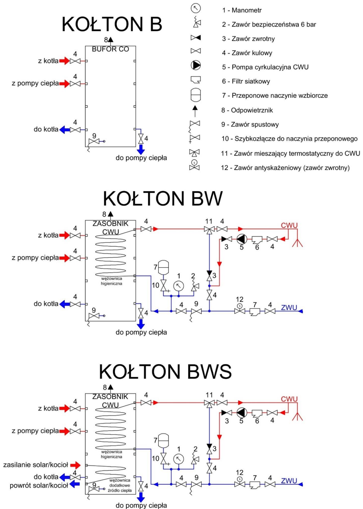
Rysunek 1. Zbiorniki buforowe Kołton
