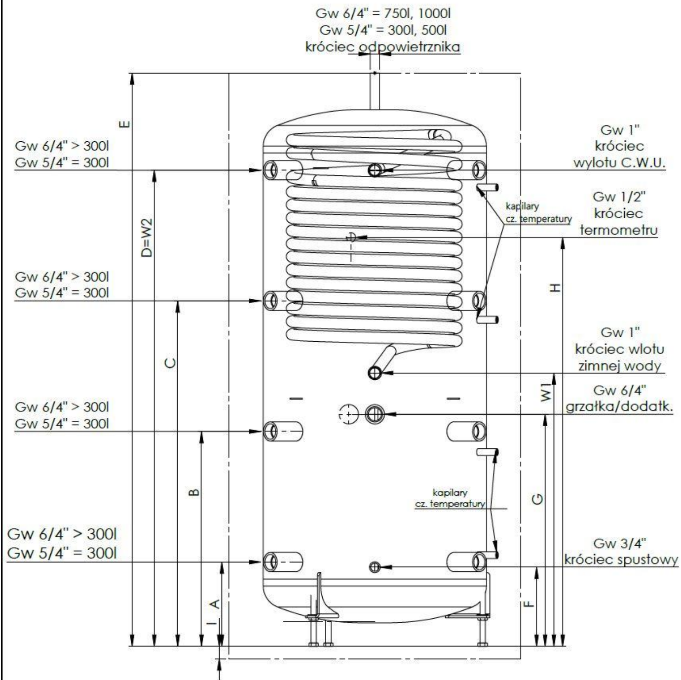
Rysunek 5. Zbiornik buforowy seria BW z wężownicą higieniczną
