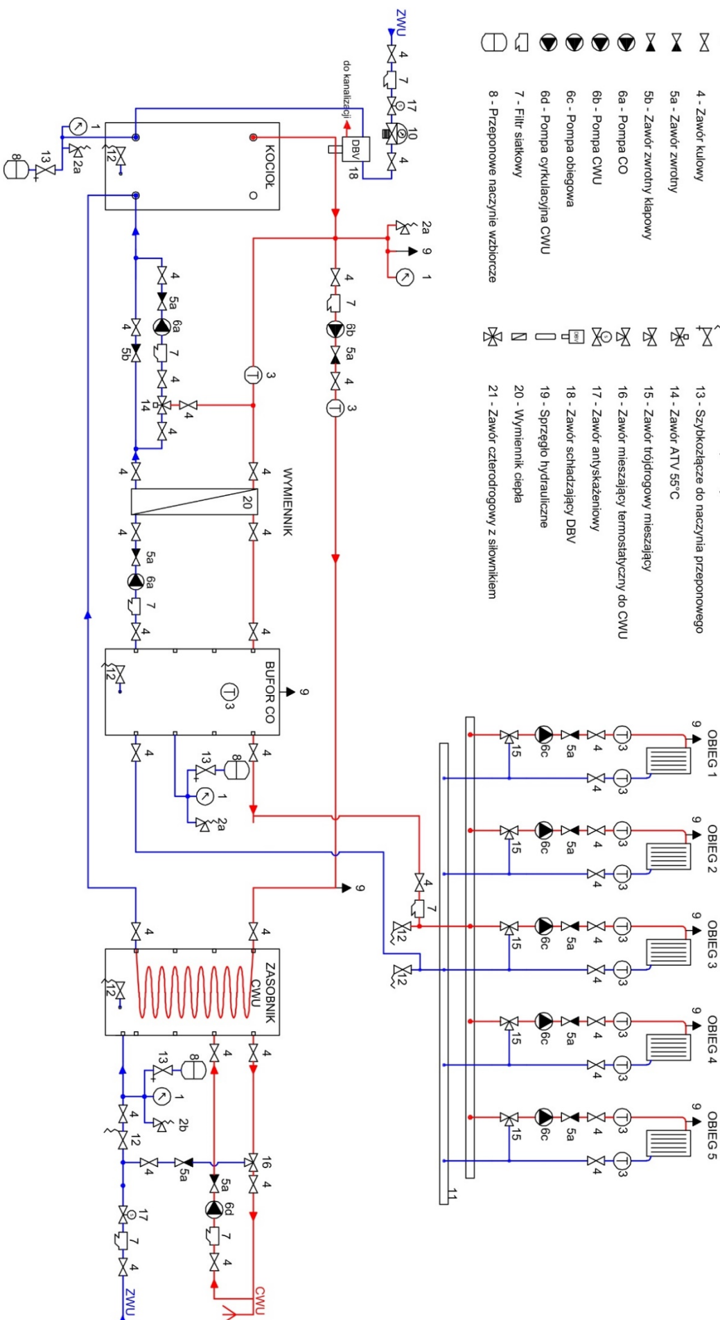
Rysunek 11. Schemat 5. KOCIOŁ + WYMIENNIK POŚREDNI + BUFOR + CWU z kotła
