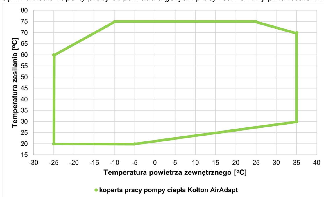
Rysunek 1. Koperta pracy pompy ciepła.
