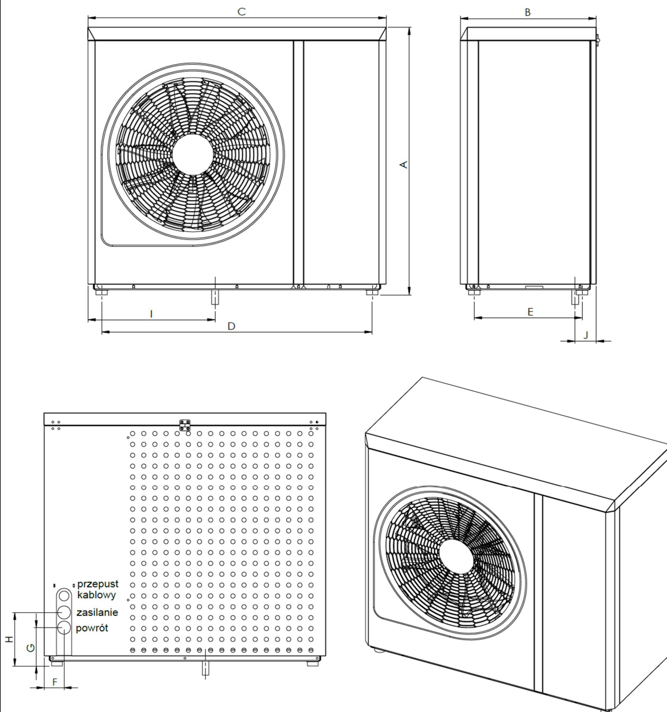
Rysunek 4. Wymiary pomp ciepła AirAdapt wraz z odpływem skroplin i postumentem [mm].
