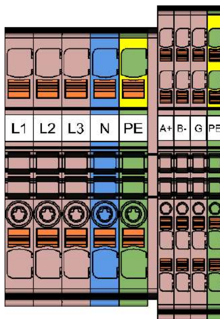
Rysunek 11. Schemat złączek w pompie ciepła AirAdapt.
