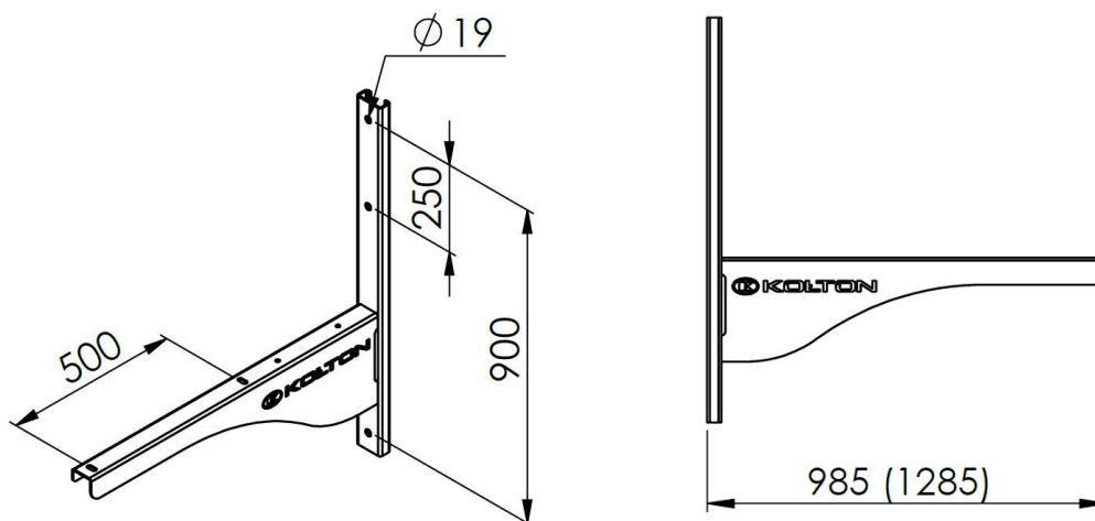
Rysunek 5. Podpory metalowe dostępne u producenta.
